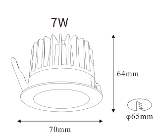
YND-F25-7W
